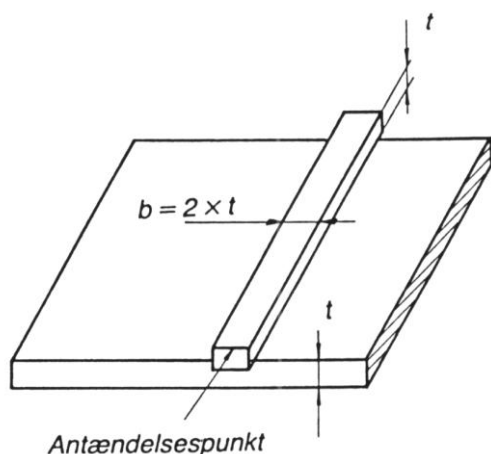
Strimmelladning på stålplade
