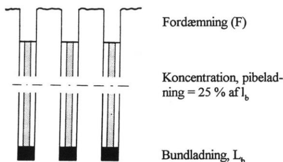
Ladningernes fordeling i borehul.
