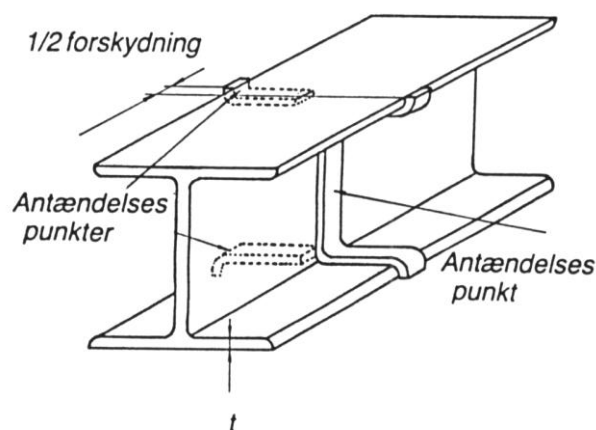
Strimmelladning på stålprofil
