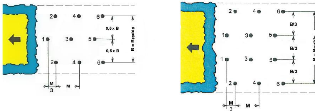
Boremønstre ved almindelig rørgravssprængning.
